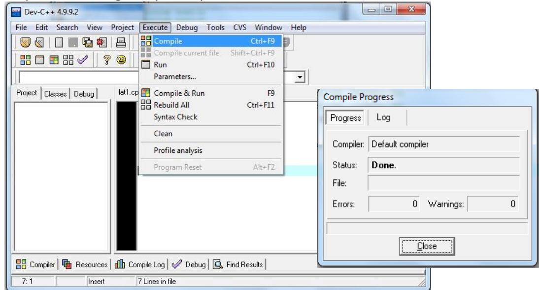
Gambar 1.6 Menterjemahkan/compile program
