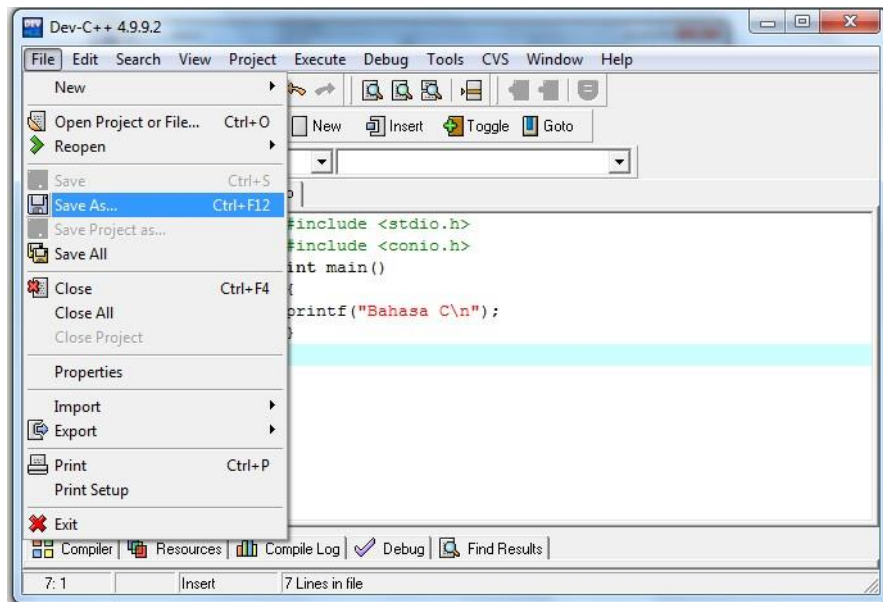
Gambar 1.5 menyimpan file
