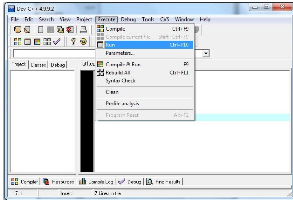
Gambar 1.7 Menjalankan program
